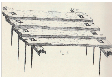
Aufbau des Bohlen- und Pfahlwegs
